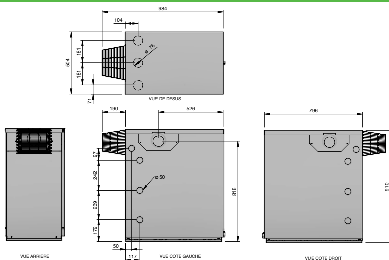
Dimensions chaudières Vortex Outdoor Bas NO x 18 kW et 24 kW
